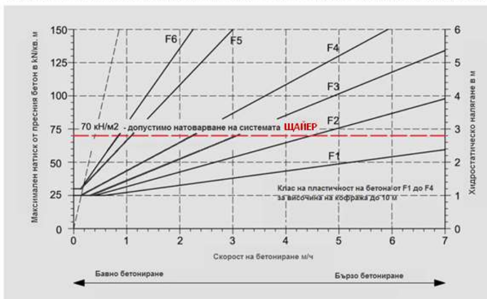
Диаграма за зависимостта на максималната скорост на бетониране от консистенцията на бетона
